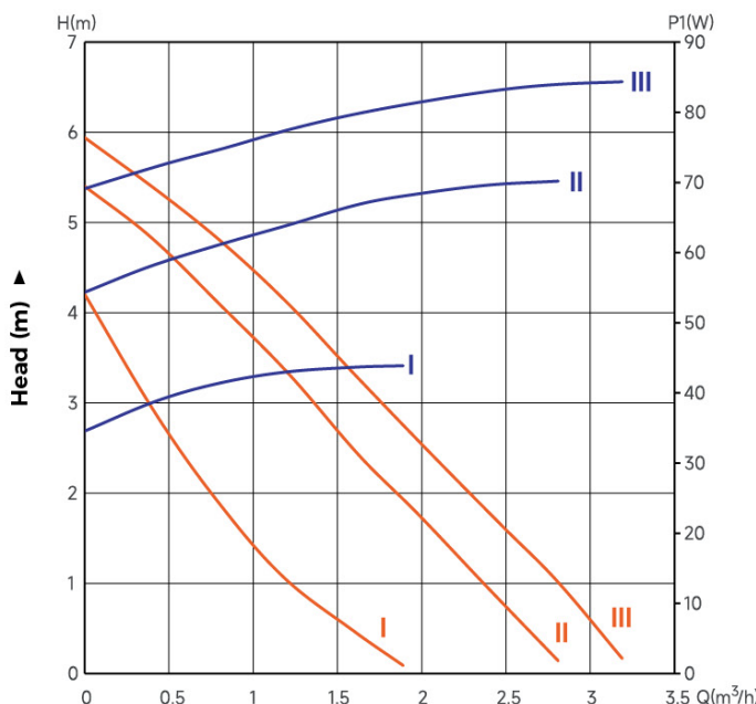
Capacity Q ► LRP20-60/130 — Q-P — Q-H
