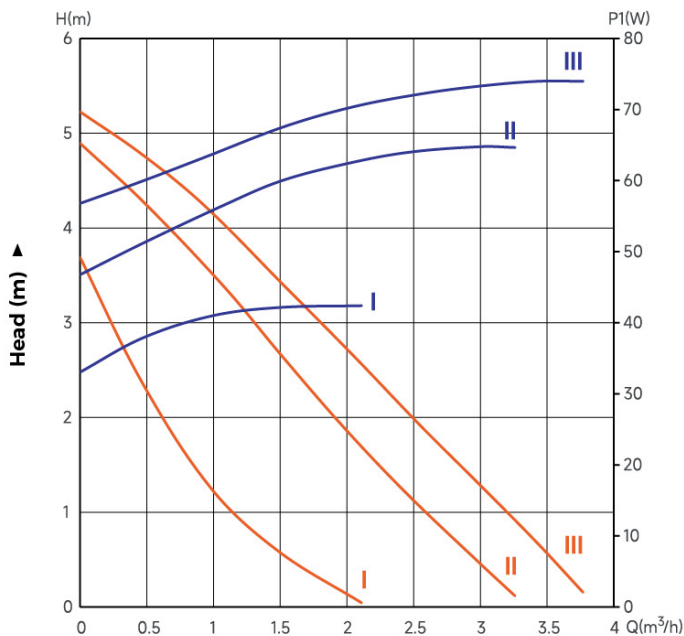
Capacity Q ► LRP32-50/180 — Q-P — Q-H
