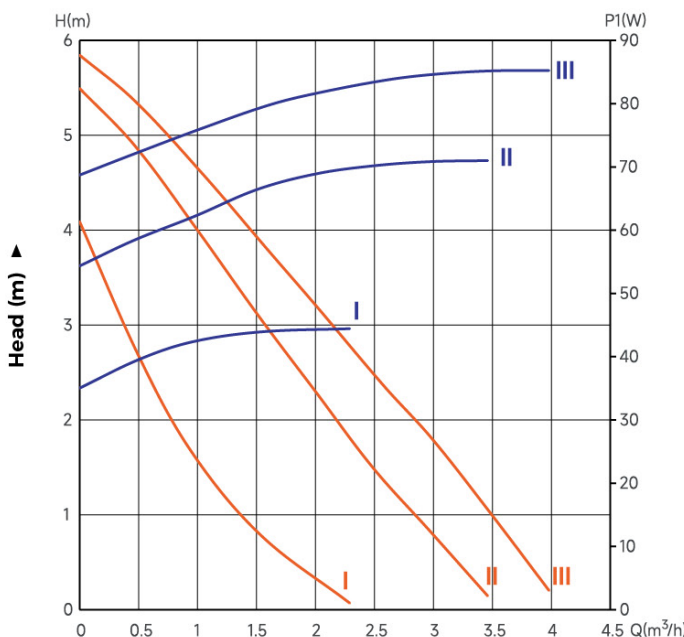
Capacity Q ► LRP32-60/180 — Q-P — Q-H
