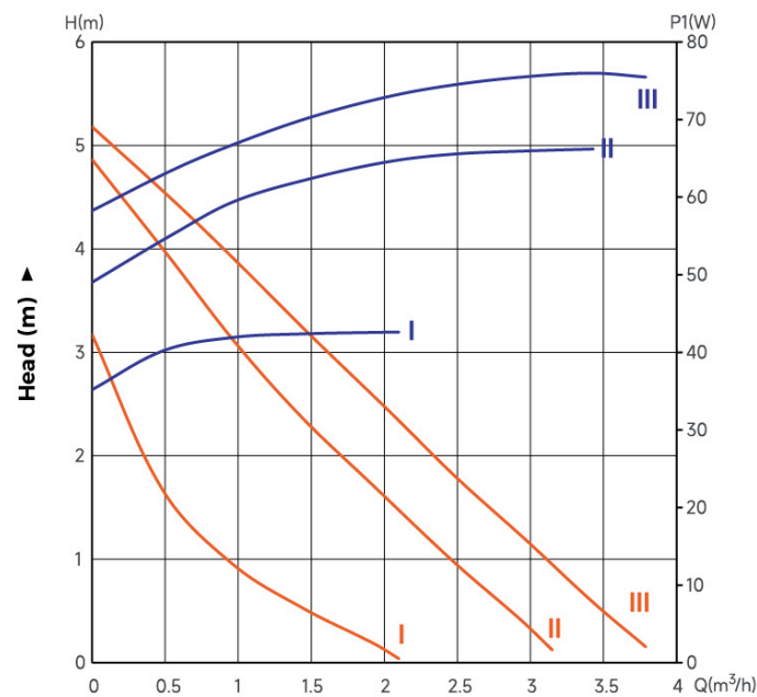
Capacity Q ► LRP25-50/180 — Q-P — Q-H
