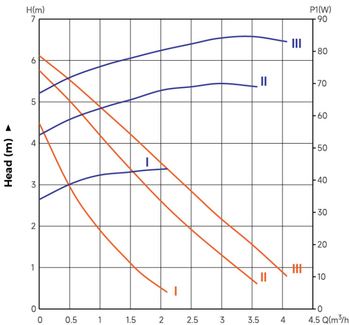
Capacity Q ► LRP25-60/180 — Q-P — Q-H
