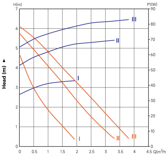
Capacity Q ► LRP25-60/130 — Q-P — Q-H
