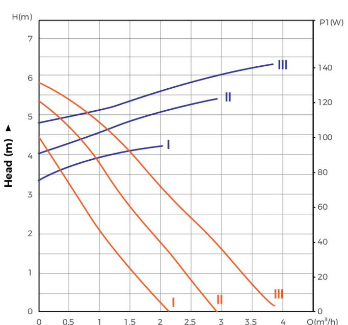
Capacity Q ► LRP25-70/130 — Q-P — Q-H
